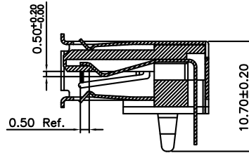
SEC:A-A
